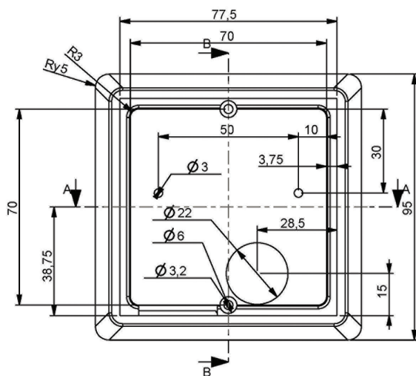
Boîtier IHM vue de face et vue de côté
