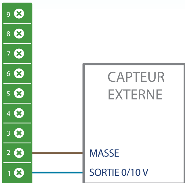
- Figure 6 Exemple de connections avec des capteurs externes -
