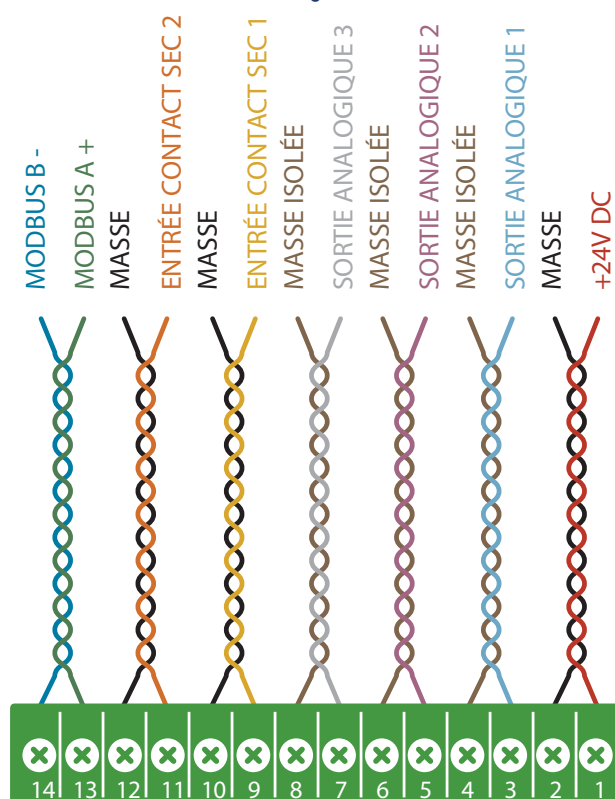
CONNECTEUR (A) AFX9
